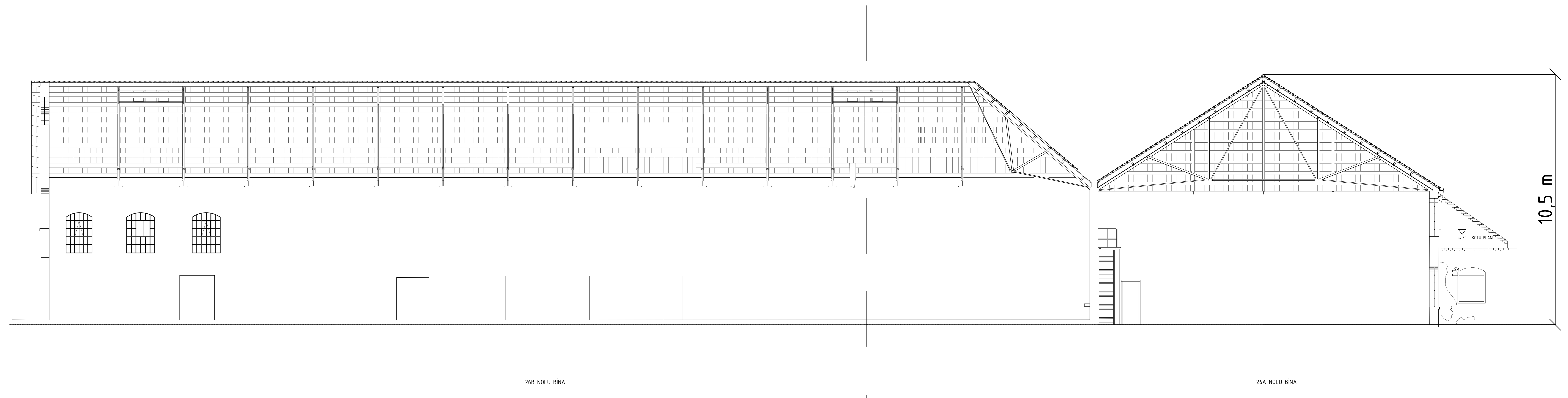
A-A KESITI
